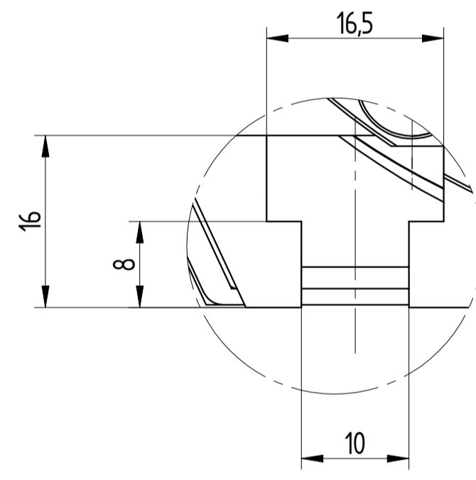
DETTAGLIO A 2:1
